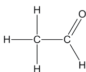
etanal
