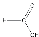
kyselina metanová
