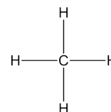
metan
