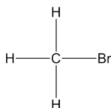
brommetan
