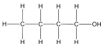
butan-1-ol
