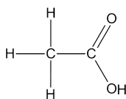
kyselina etanová
