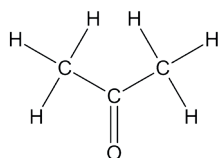
dimetylketon
