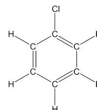
chlorbenzen
