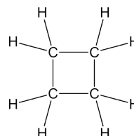
cyklobutan
