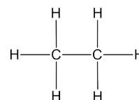
etan
