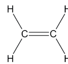
eten
