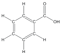
kyselina benzoová
