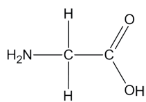
kyselina aminoetanová
